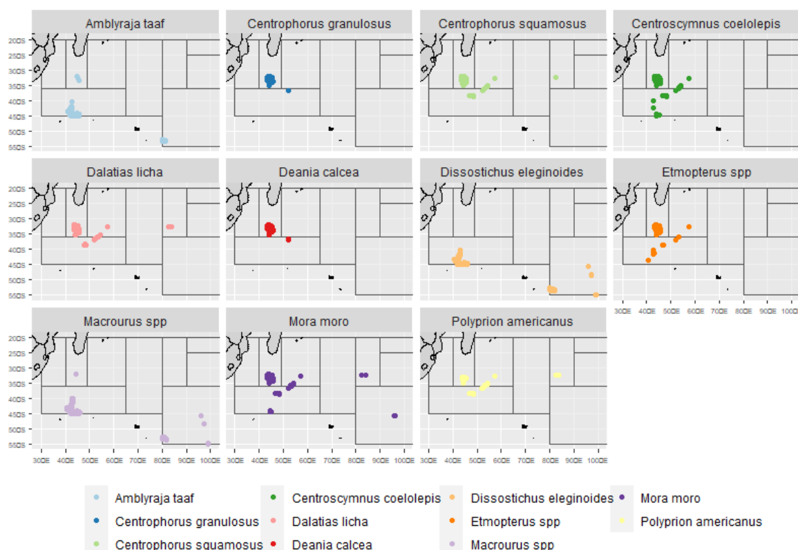
Figura 6. Distribución del bycatch en las pesquerías españolas de palangre de fondo en el área de SIOFA. Fuente: Rueda et al. (2023).
