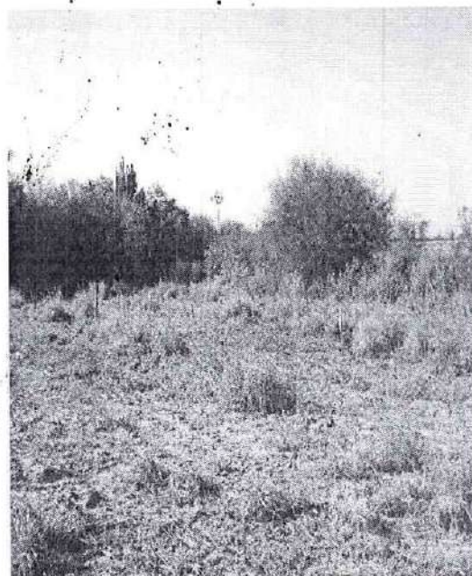
Imagen N° 18. Parcela Cambisol
